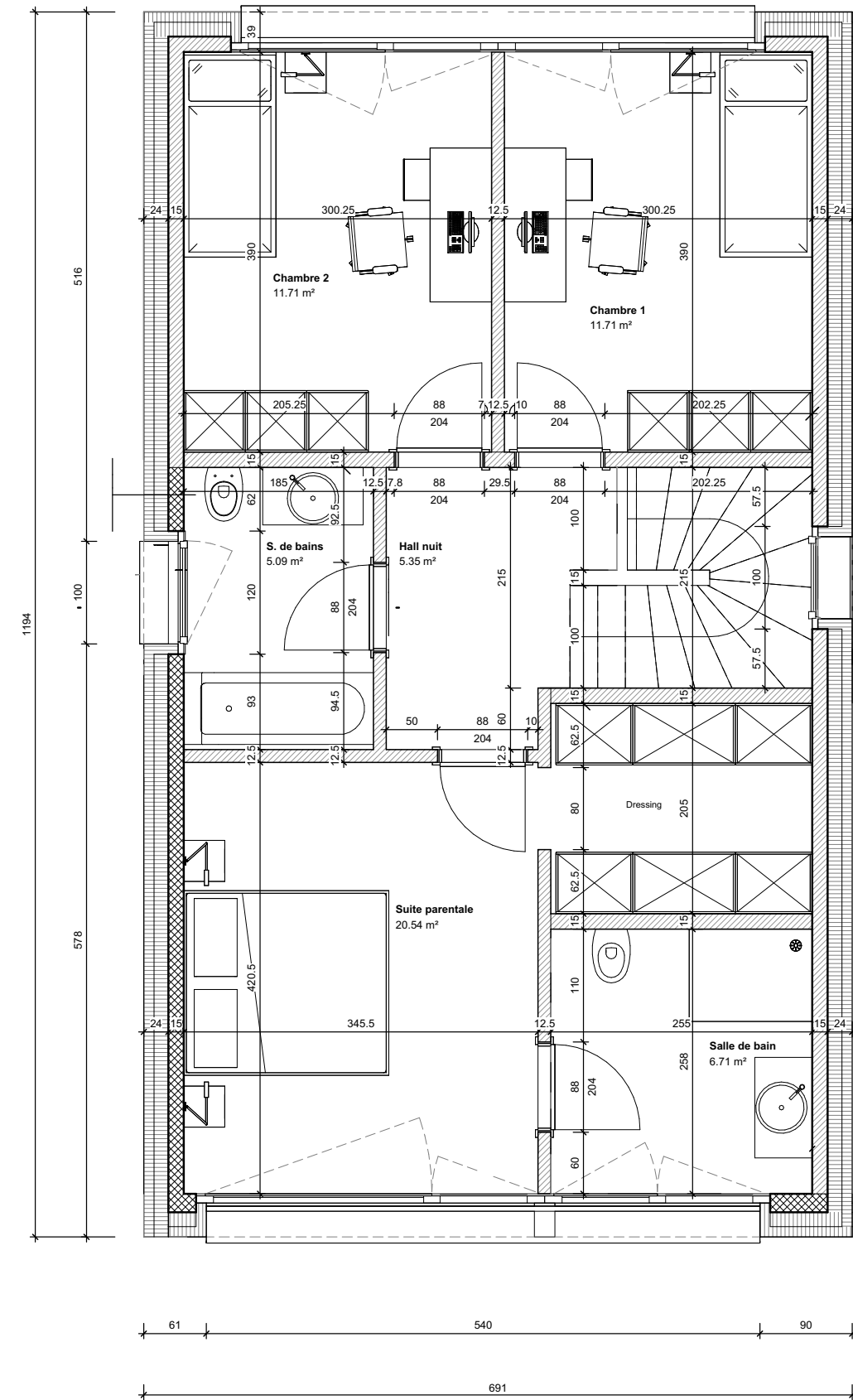
ETAGE
